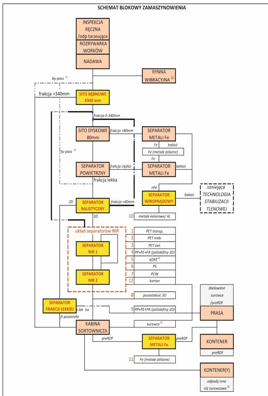
Rysunek 8 Schemat blokowy zamaszynowania – przykładowe rozwiązanie
