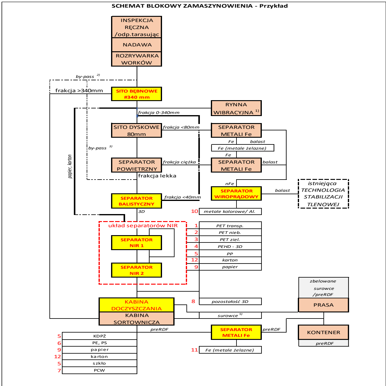
Rysunek 8 Schemat blokowy zamaszynowania – przykładowe rozwiązanie
